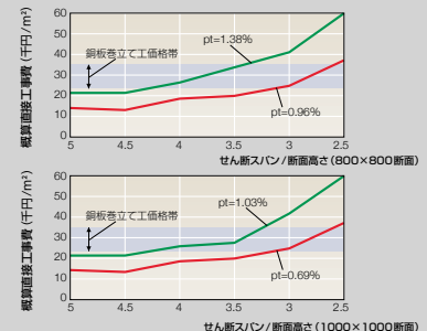
・A&P耐震補強工法の概算直接工費と「せん断スパン/断面高さ」の関係
