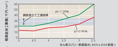
・A&P耐震補強工法の概算直接工事費と「せん断スパン/断面高さ」の関係
