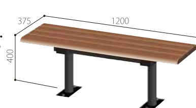
品番：DLB-90*40R-FLAT*1200-BP サイズ：W375×L1200×H400 標準価格 78,200円 / 基(税抜)
