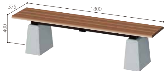
品番：DLB-90*40R-FLAT-PC サイズ：W375×L1800×H400 標準価格 90,000円 / 基(税抜)
