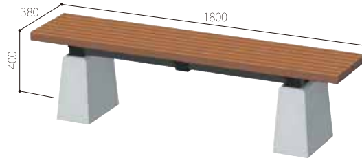
品番：DLB-50*45-FLAT-PC サイズ：W380×L1800×H400 標準価格 135,000円 / 基(税抜)
